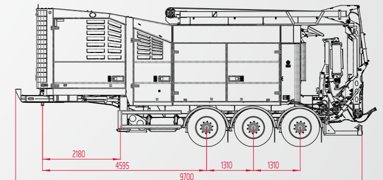
Seitenansicht:
