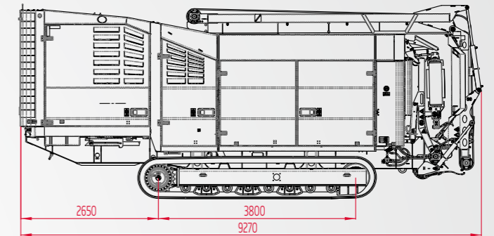
Seitenansicht:
