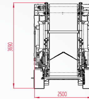
Rückansicht:
